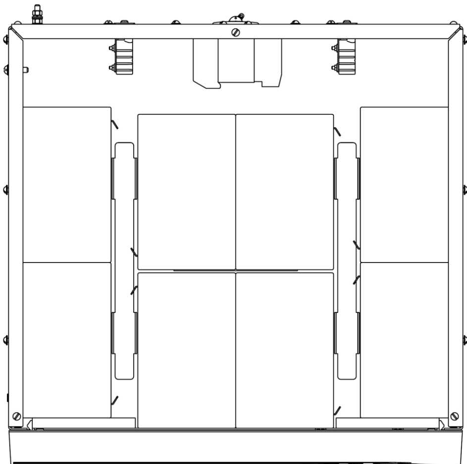
Рисунок 3 – Размещение аккумуляторных батарей в корпусе
