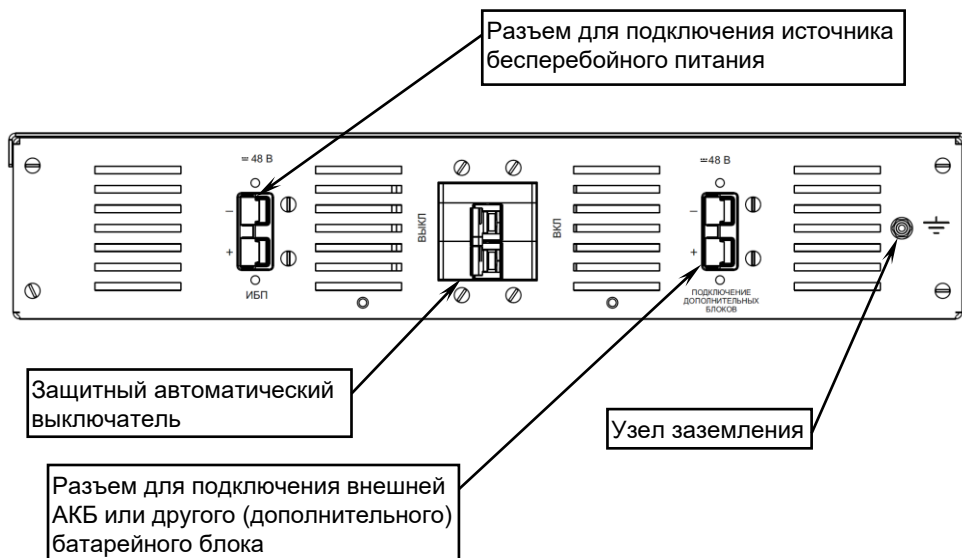
Рисунок 2 – Общий вид задней панели изделия со снятыми заглушками разъемов
