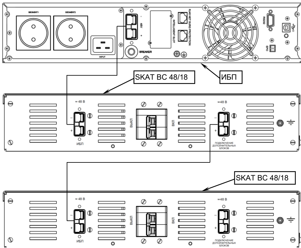
Рисунок 5 — Подключение ИБП и дополнительного батарейного блока
