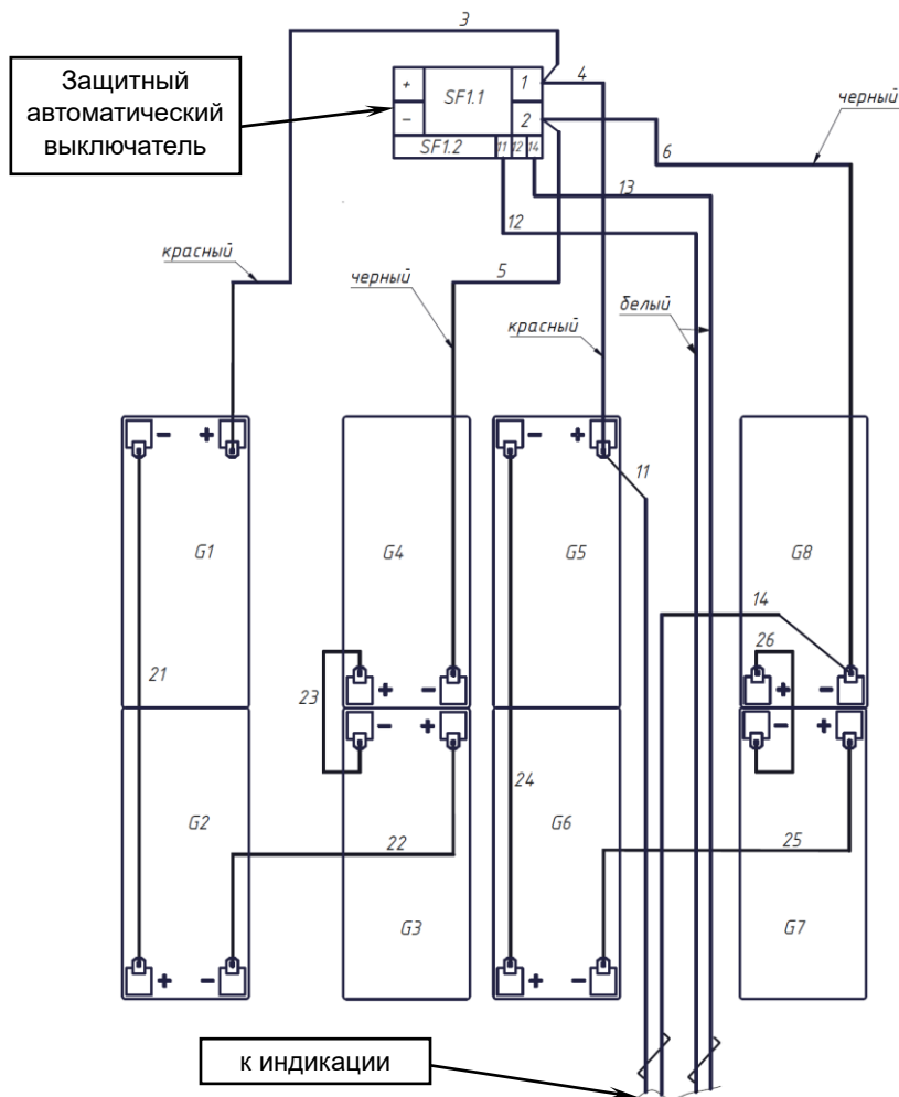
Рисунок 7 — Схема соединений аккумуляторных батарей
