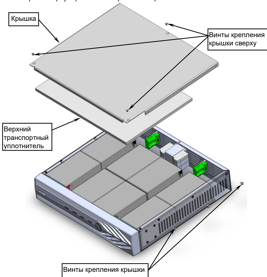
Рисунок 6 — Замена аккумуляторных батарей.
