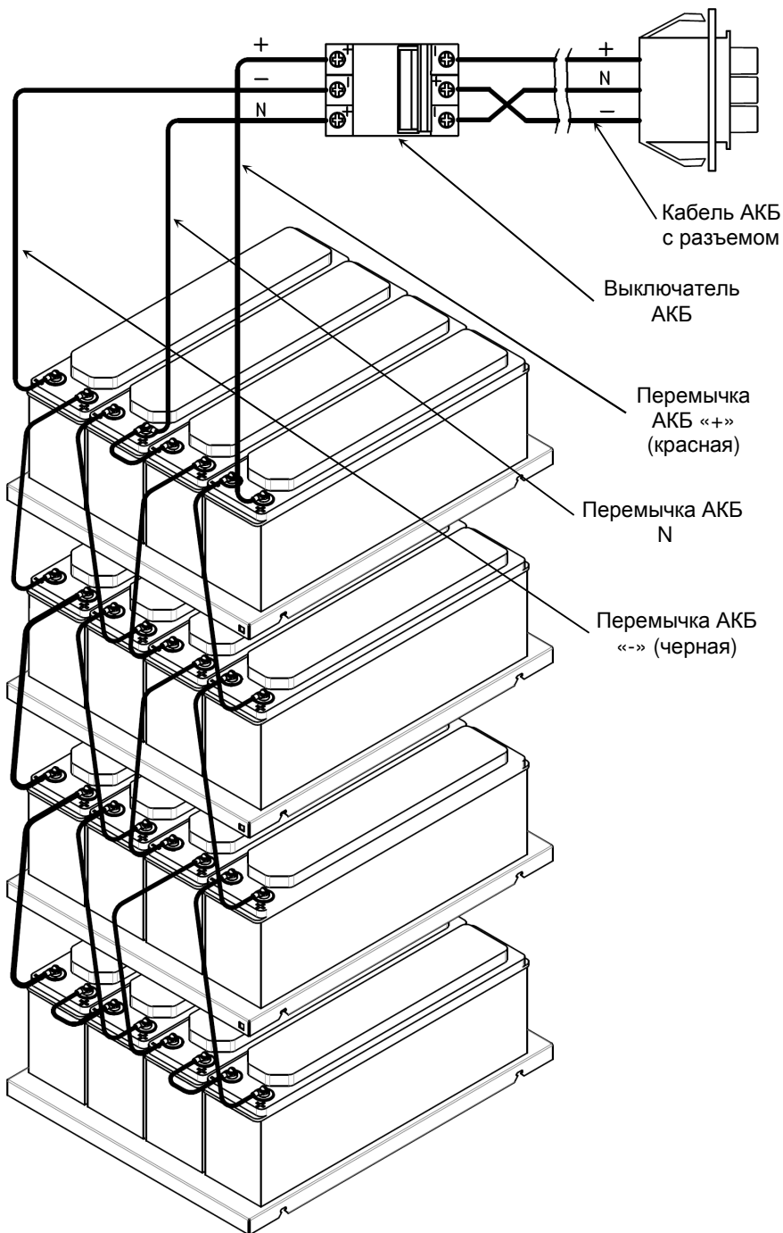
Рисунок 4 — Пример размещения и подключения на полках комплекса.
