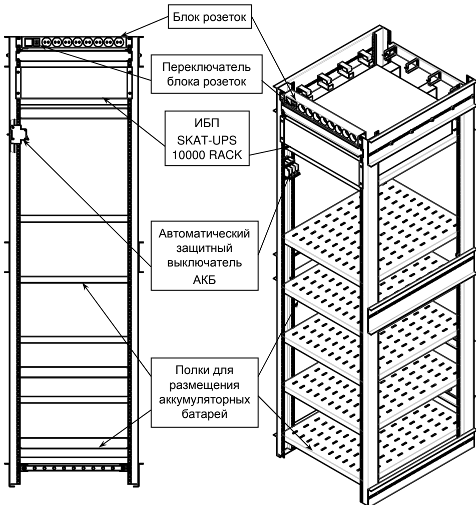
Рисунок 1 — Общий вид изделия спереди, без оболочки.
