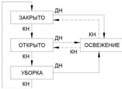
Рисунок 2 - схема управления модулем с помощью кнопки. КН - короткое нажатие, ДН - длительное нажатие.
