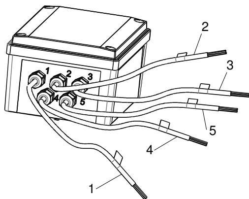
Рисунок 2 – Маркировка кабелей
