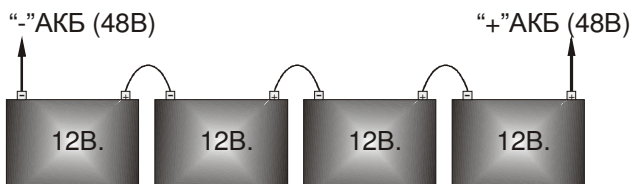
Схема соединения аккумуляторных батарей
