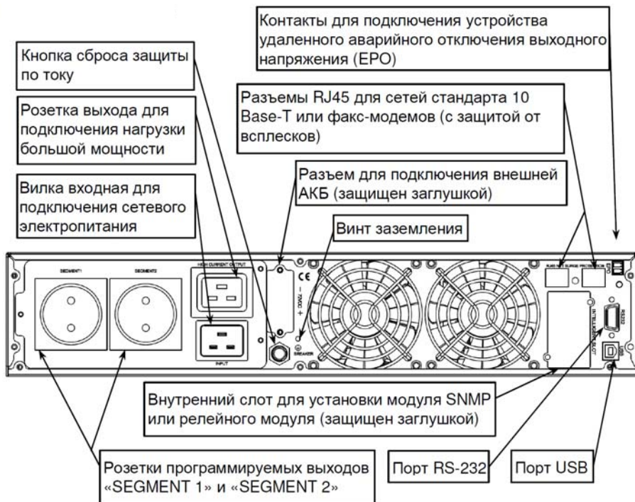
Рисунок 5 — общий вид задней панели ИБП.
